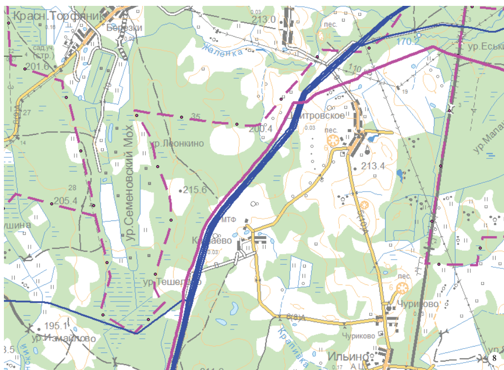
ВЛ-10 кВ
