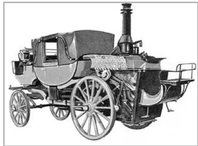
«Паровые экипажи» активно разрабатывались во 2-й половине XIX века во всех странах Европы. Паровая карета Б. Вирджинию. 1854 год
